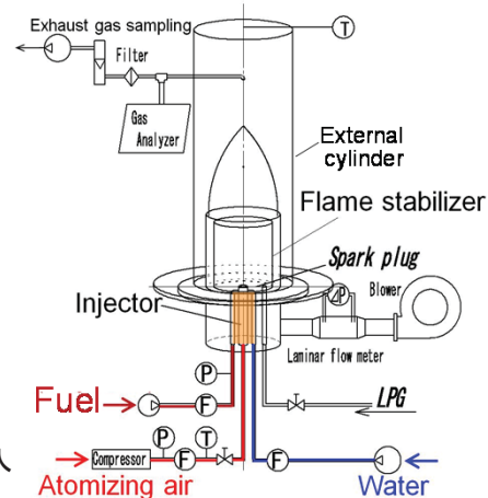
図3 バーナー燃焼試験装置
